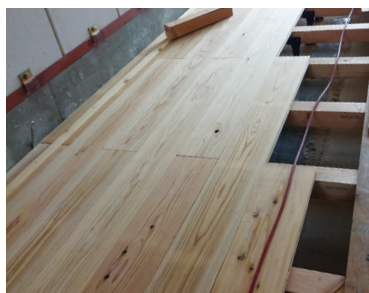
大引(米松KD 90角)に直接施工
